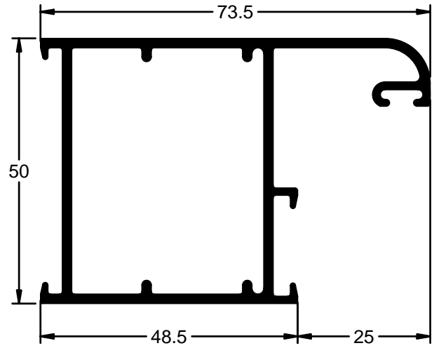
CERCO PARA FIJOS
