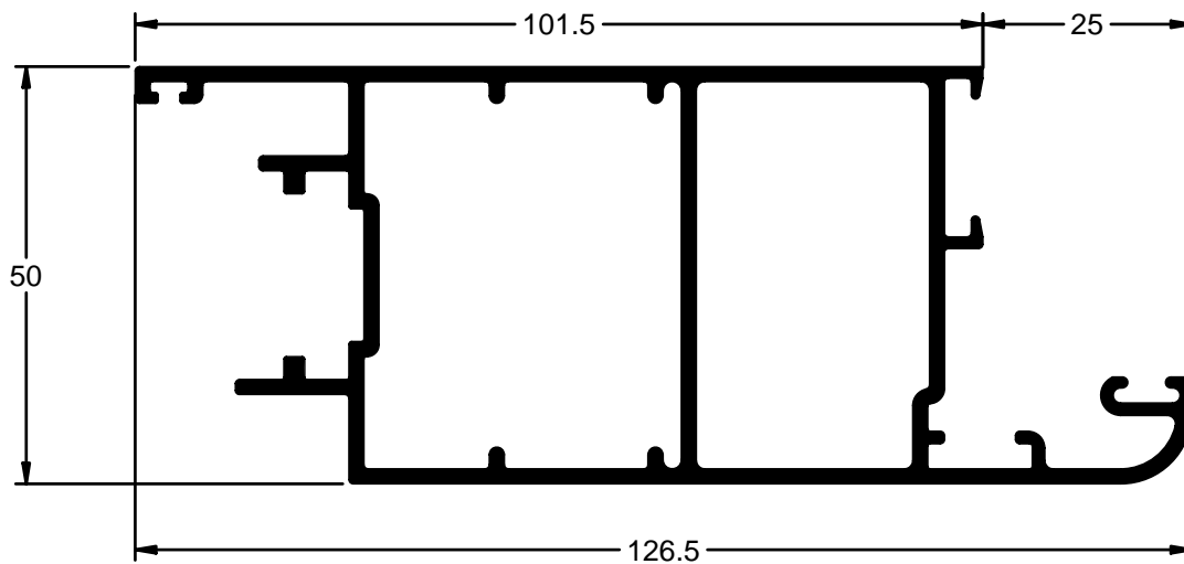
HOJA APERTURA INTERIOR
