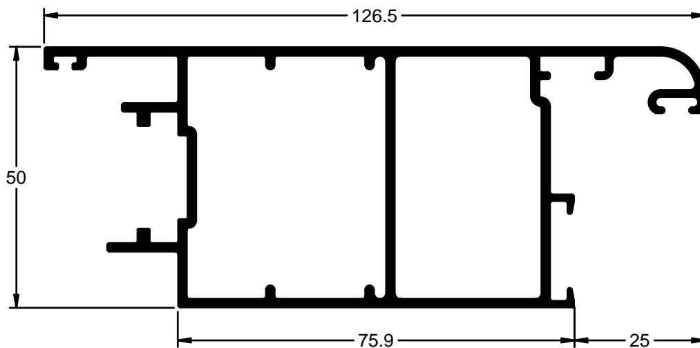
HOJA APERTURA EXTERIOR
