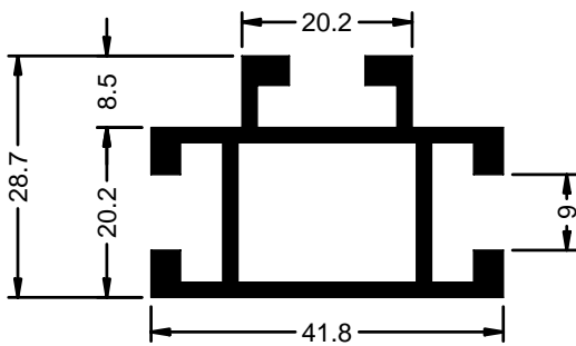
TRAVESAÑO 3 RANURAS
