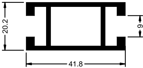
TRAVESAÑO 2 RANURAS
