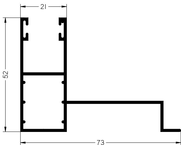
MAINEL MONOBLOCK
