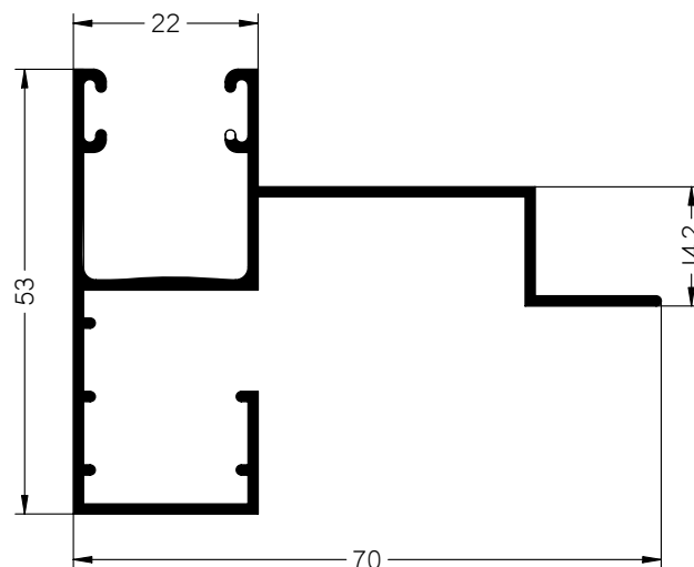
MAINEL MONOBLOCK
