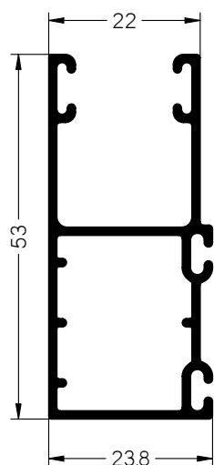
MAINEL 2 PIEZAS
