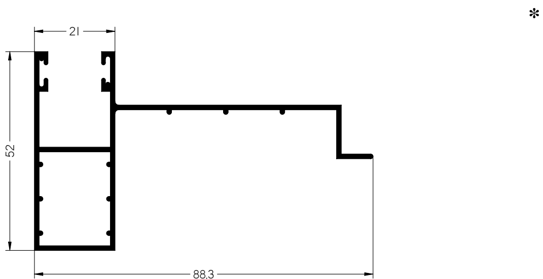
MAINEL MONOBLOCK
