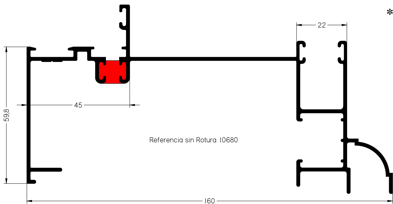
MAINEL MONOBLOCK
