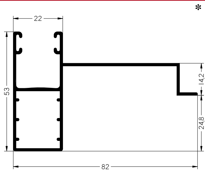
MAINEL MONOBLOCK
