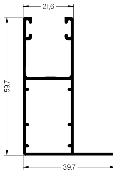
MAINEL MONOBLOCK
