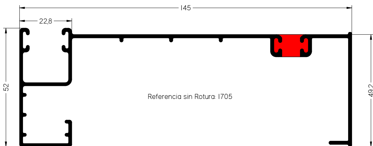
MAINEL MONOBLOCK
