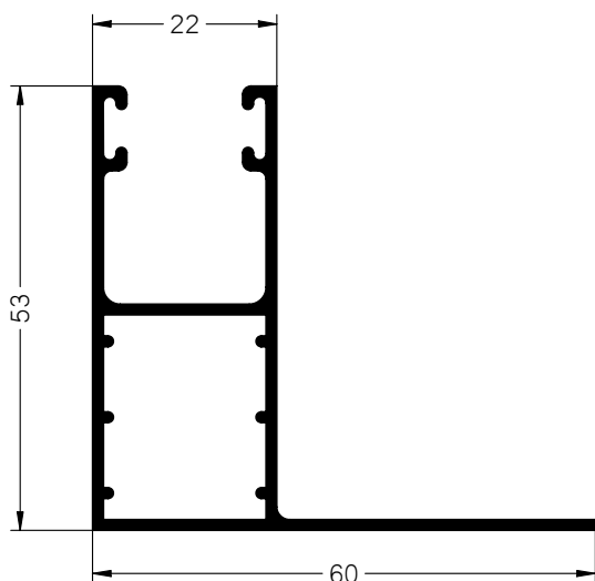
MAINEL MONOBLOCK
