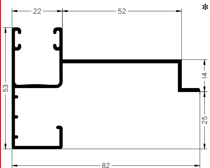
MAINEL MONOBLOCK
