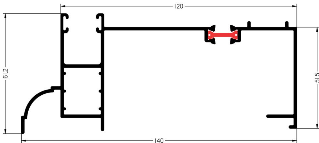
MAINEL MONOBLOCK
