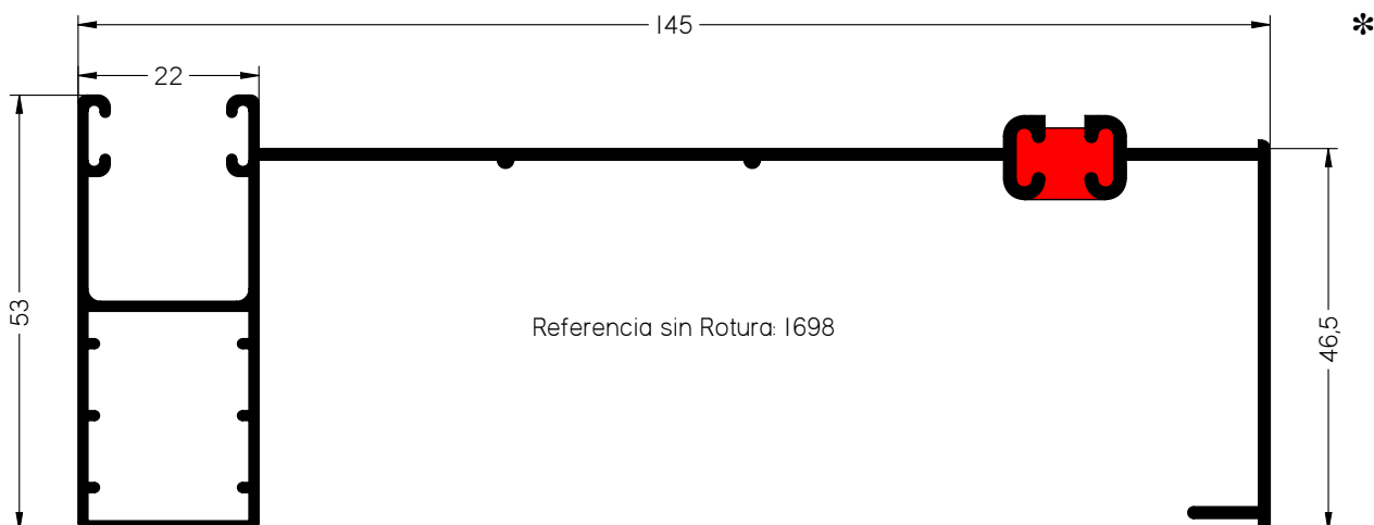
MAINEL MONOBLOCK
