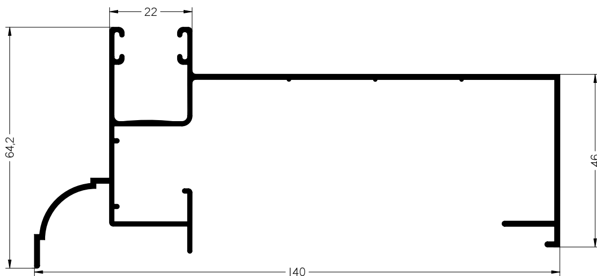
MAINEL MONOBLOCK
