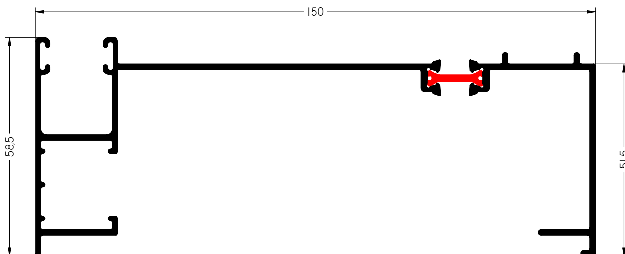
MAINEL MONOBLOCK
