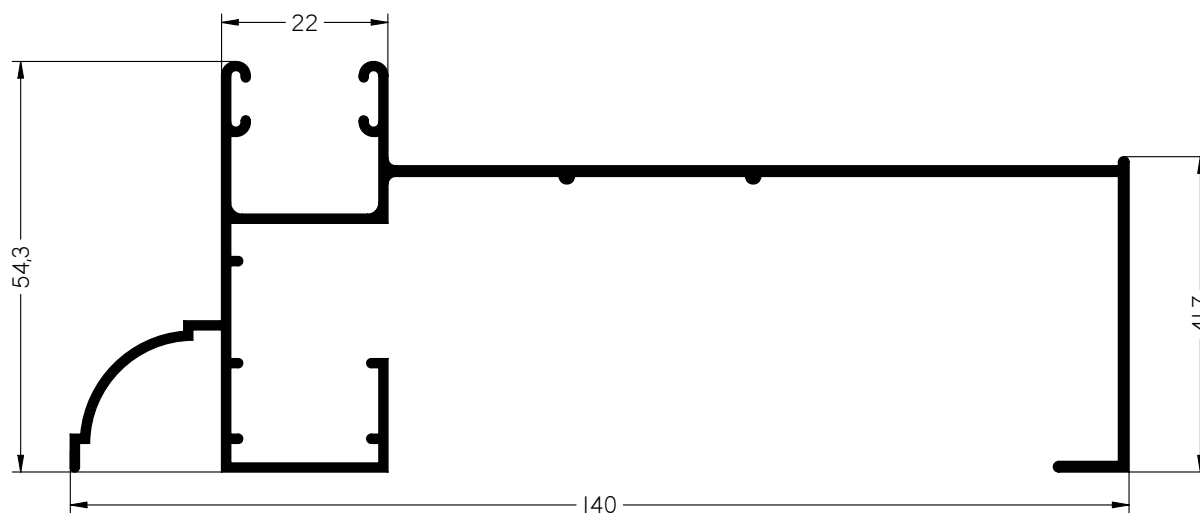
MAINEL MONOBLOCK
