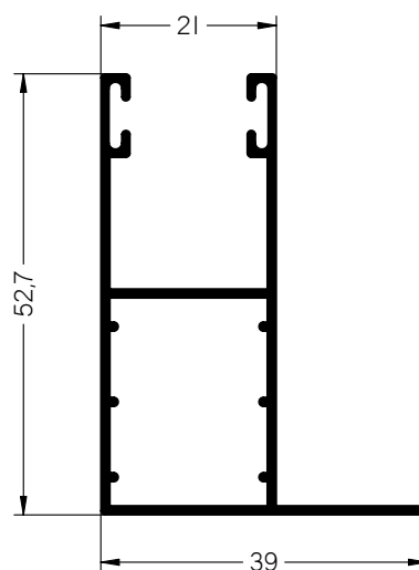
MAINEL MONOBLOCK
