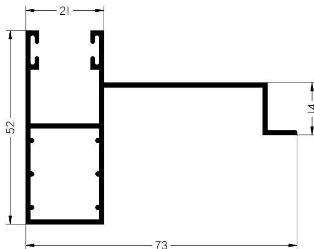
MAINEL MONOBLOCK
