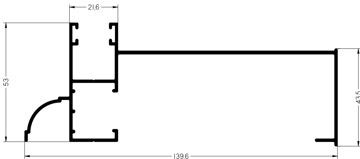
MAINEL MONOBLOCK
