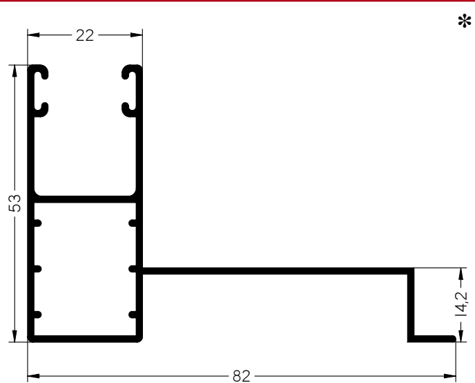
MAINEL MONOBLOCK
