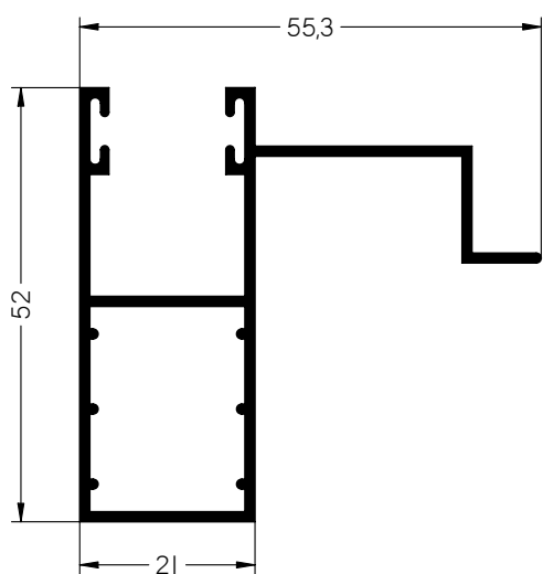
MAINEL MONOBLOCK
