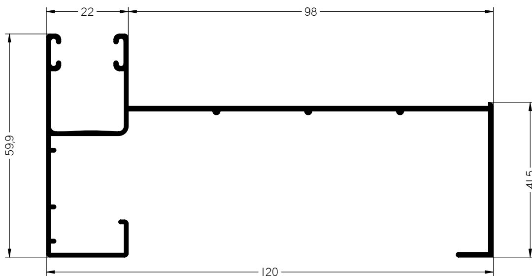
MAINEL MONOBLOCK
