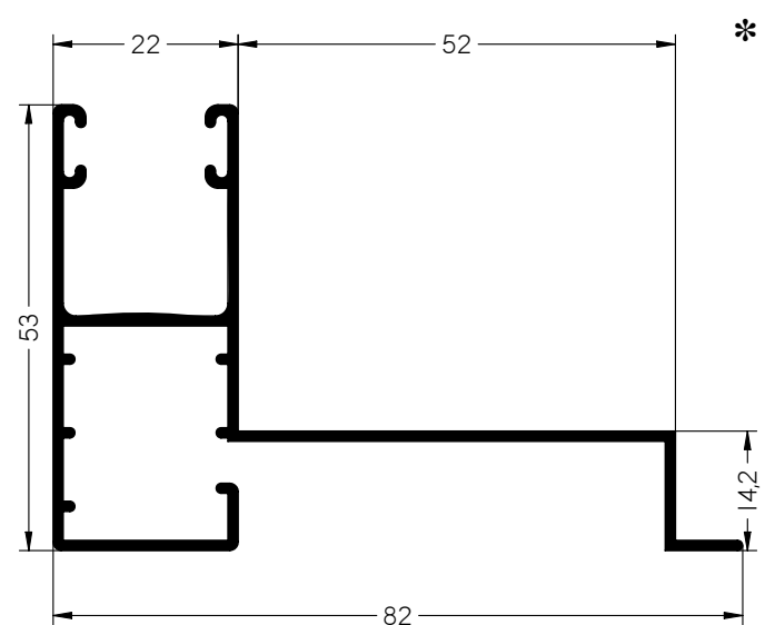
MAINEL MONOBLOCK
