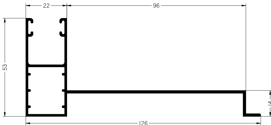
MAINEL MONOBLOCK
