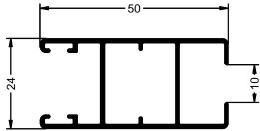
HOJA LATERAL
