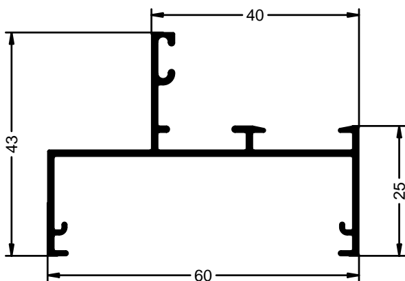
CERCO FIJO
