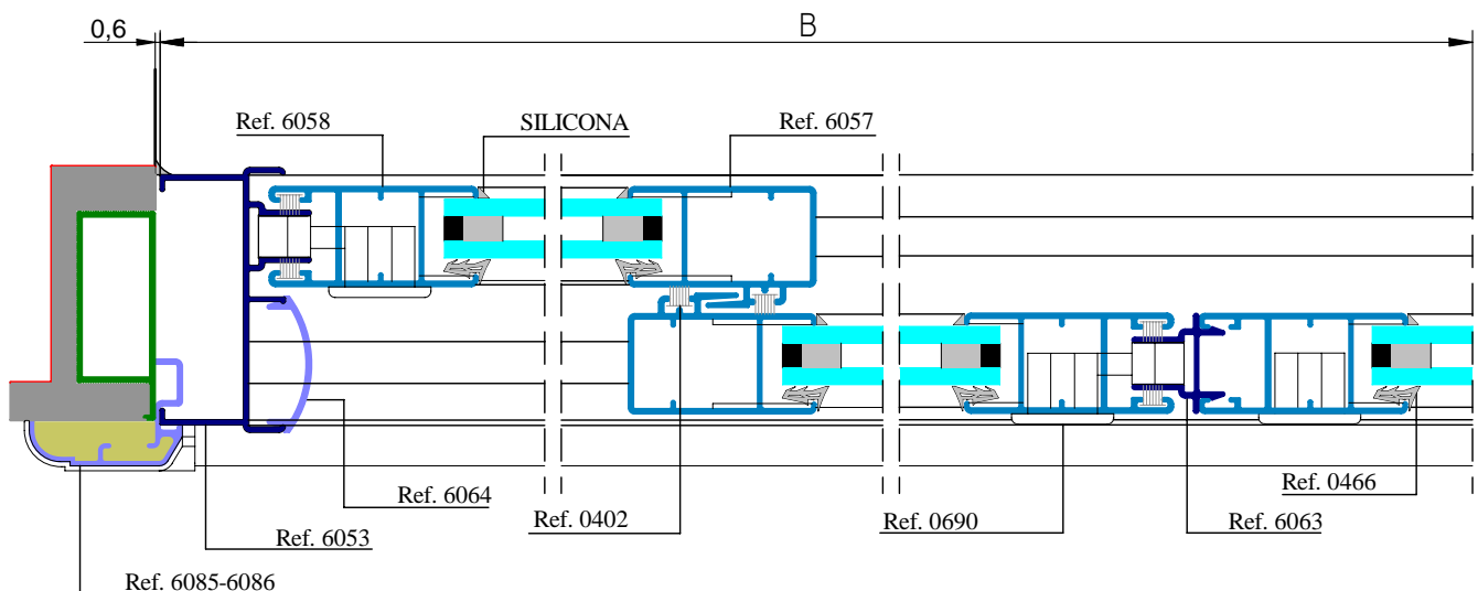
SECCION HORIZONTAL
