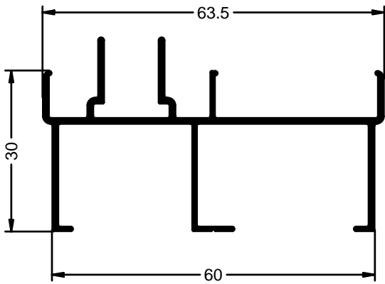
CERCO LATERAL
