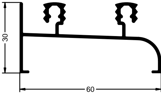
CERCO INFERIOR
