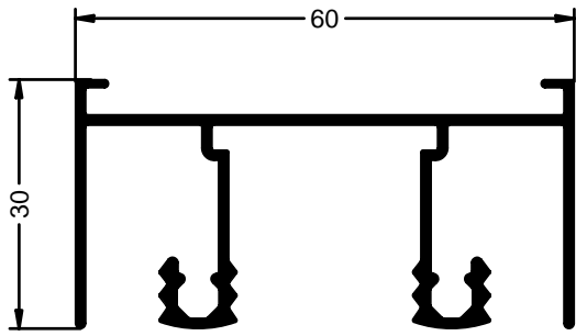
CERCO SUPERIOR
