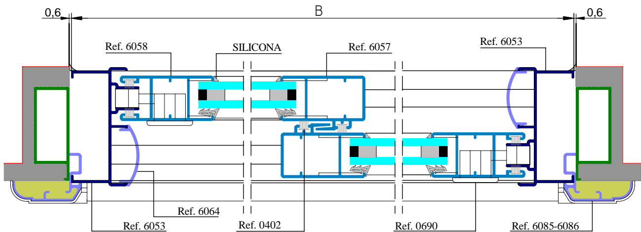
SECCION HORIZONTAL
