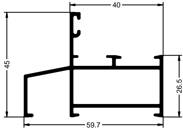
CERCO FIJO
