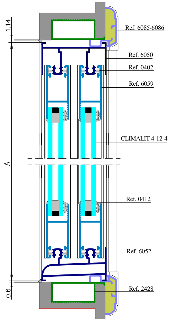
SECCION VERTICAL
