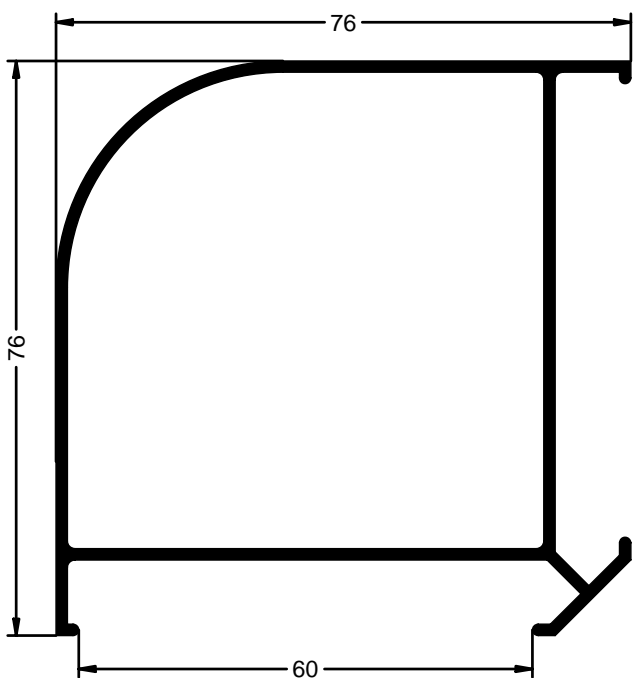
ESQUINERO REDONDO
