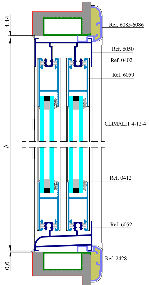
SECCION VERTICAL
