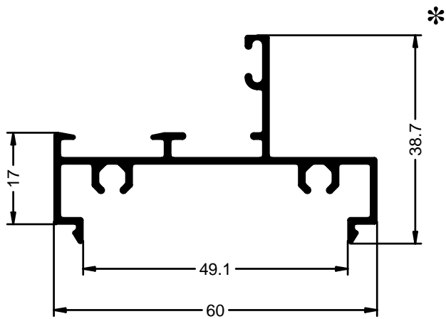
CERCO FIJO
