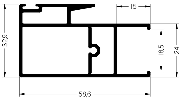
HOJA CENTROS CLIMALIT
