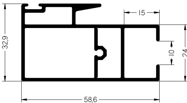
HOJA CENTROS CRISTAL MONOLITICO
