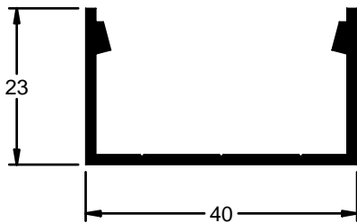
ANCLAJE BARANDILLA
