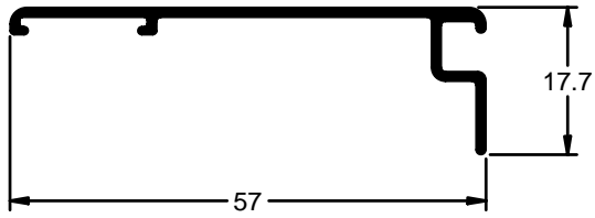
SOLAPE DE 57mm
