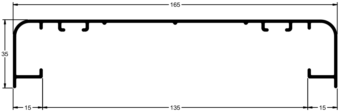
ALBARDILLA DE 165
