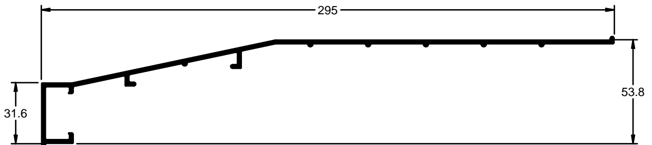
ALFEIZAR DE 295mm
