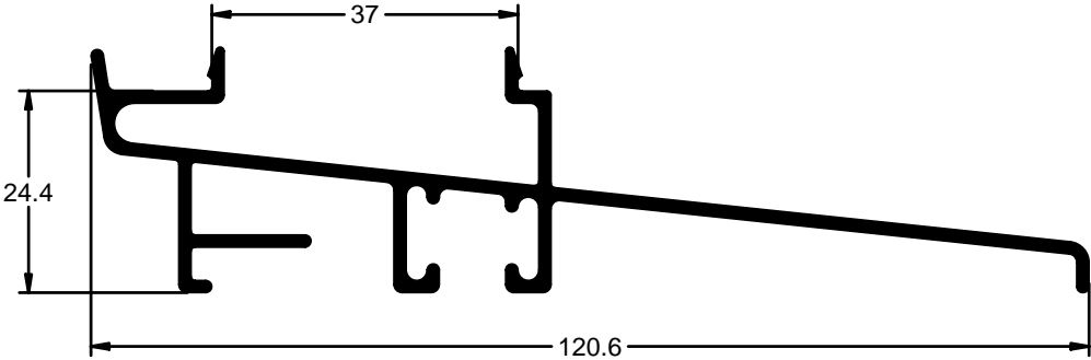
PERFIL CONDENSACION S/EUROTHERMIC
