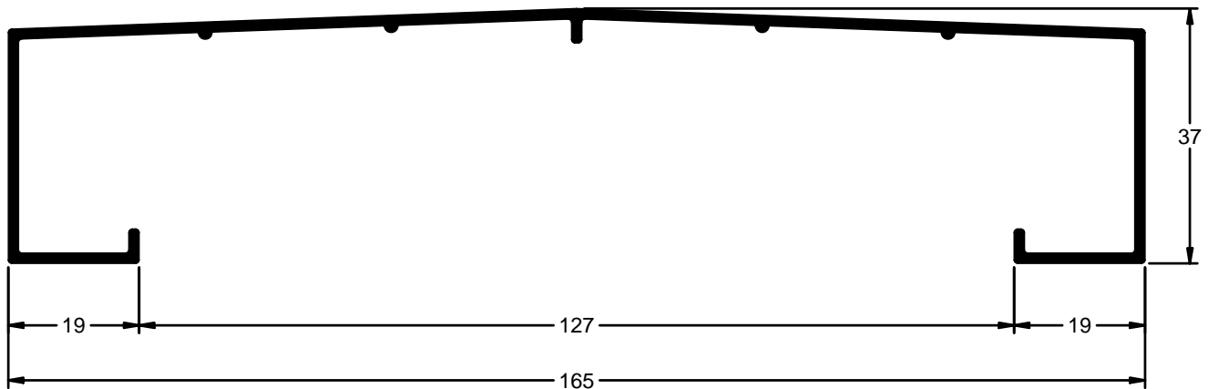
ALBARDILLA DE 165
