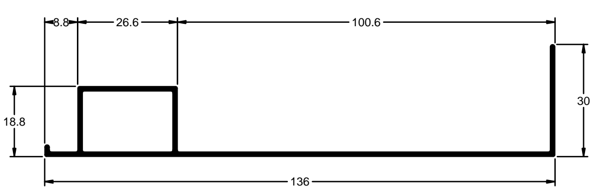
PREMARCO 136mm
